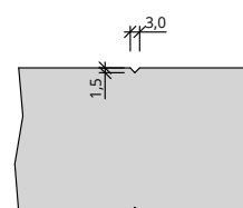
Detail Brüstungsfuge
