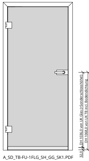
A_SD_TB-FU-1FLG_SH_GG_SK1.PDF
