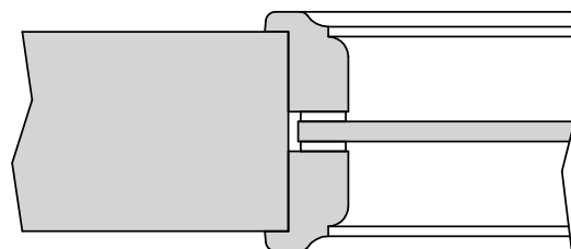
Detail Verglasung
