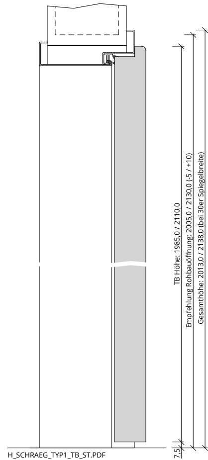
H_SCHRAEG_TYP1_TB_ST.PDF
