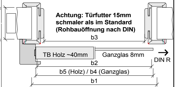
Anschlagkasten ↑ Ansichtsseite
