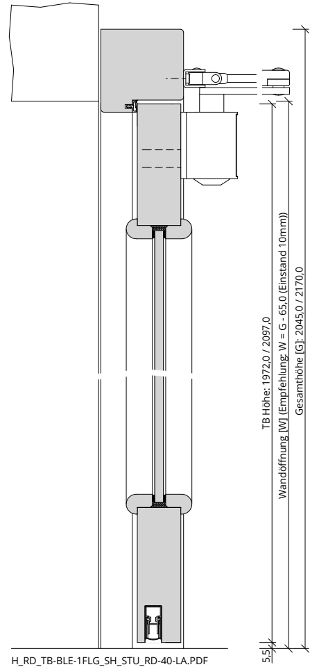
H_RD_TB-BLE-1FLG_SH_STU_RD-40-LA.PDF
