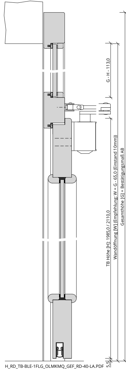
H_RD_TB-BLE-1FLG_OLMKMQ_GEF_RD-40-LA.PDF
