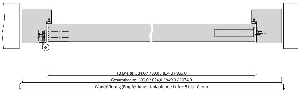
Q_RD_TB-BLO-1FLG_OLMKMQ_STU_RD-40.PDF
