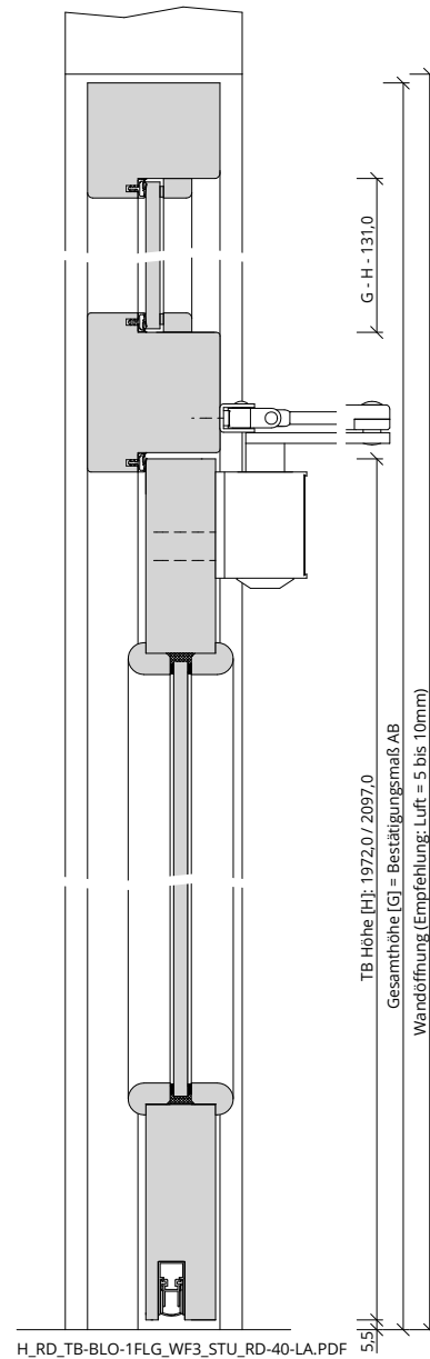
H_RD_TB-BLO-1FLG_WF3_STU_RD-40-LA.PDF
