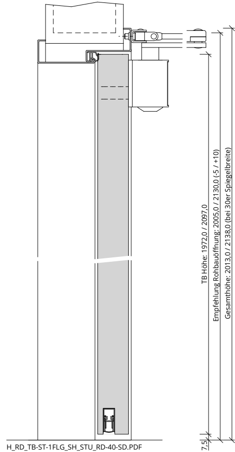
H_RD_TB-ST-1FLG_SH_STU_RD-40-SD.PDF
