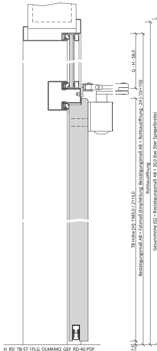
H_RD_TB-ST-1FLG_OLMKMQ_GEF_RD-40.PDF
