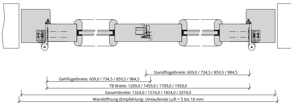
Q_RD_TB-BLO-2FLG_OBMKMQ_STU_RD-40-2-LA.PDF
