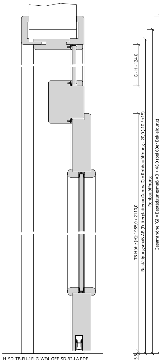
H_SD_TB-FU-1FLG_WF4_GEF_SD-32-LA.PDF
