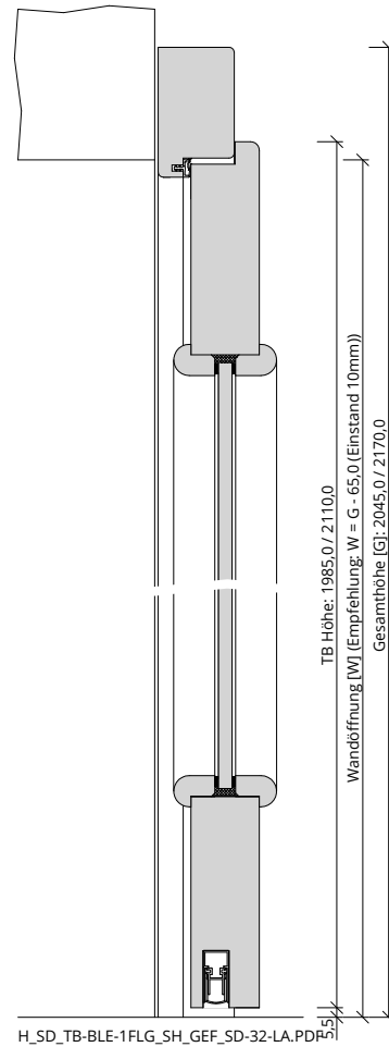
H_SD_TB-BLE-1FLG_SH_GEF_SD-32-LA.PDF
