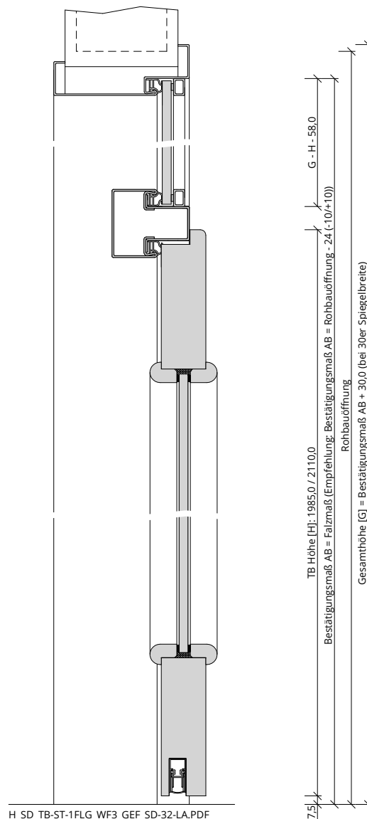
H_SD_TB-ST-1FLG_WF3_GEF_SD-32-LA.PDF
