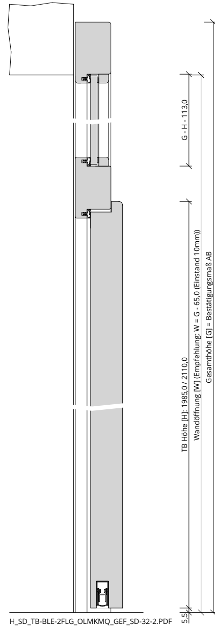
H_SD_TB-BLE-2FLG_OLMKMQ_GEF_SD-32-2.PDF
