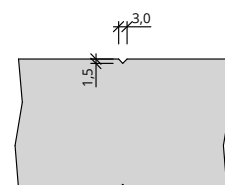
Detail Brüstungsfuge
