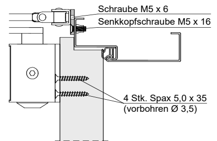
Beispiel Stahlzarge
