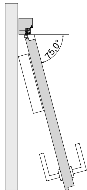
Beispiel 2: Blockrahmen – "Situation Flur" mit Standard- Türschließer
