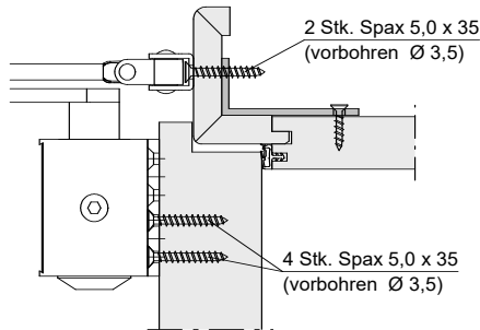
Beispiel Türfutter
